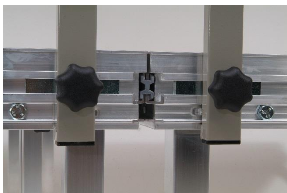
Montageschiene Detailansicht Bühnenteile mit X-Verbinder verbunden
