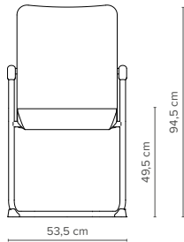
— 37/2 Tiefe 67,5 cm Gewicht 10,6 kg 4-fach stapelbar
