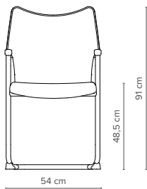
— 37/7 Tiefe 60 cm Gewicht 10,3 kg 5-fach stapelbar
